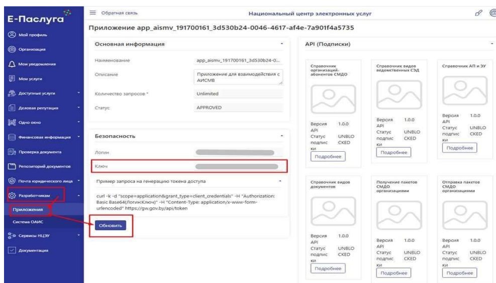
Рис. 6. Обновление ключа.
